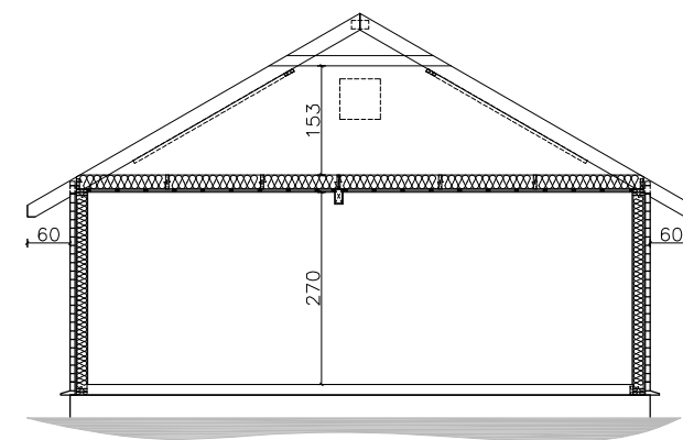
PRZEKRÓJ
