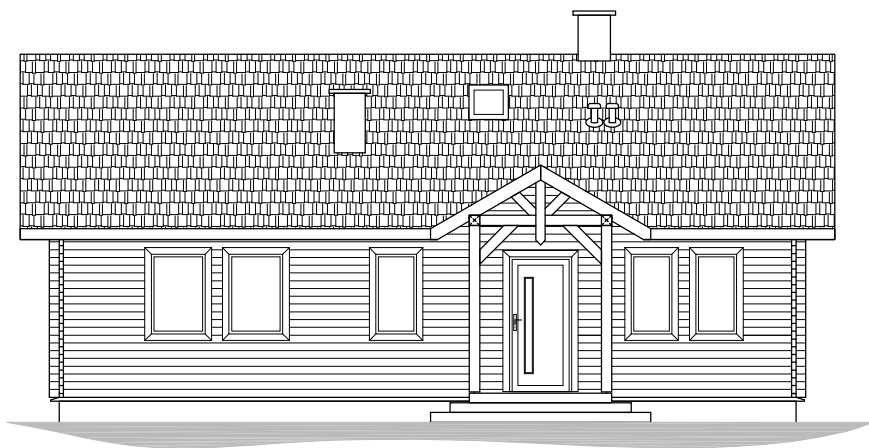
ELEWACJA FRONTOWA
