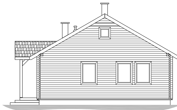
ELEWACJA BOCZNA
