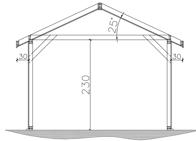
PRZEKRÓJ
