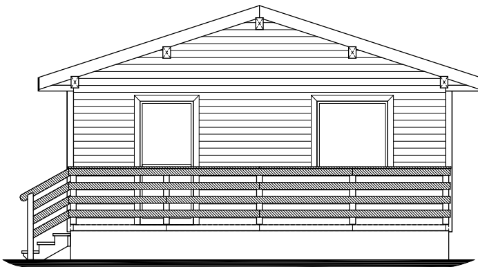
ELEWACJA FRONTOWA
