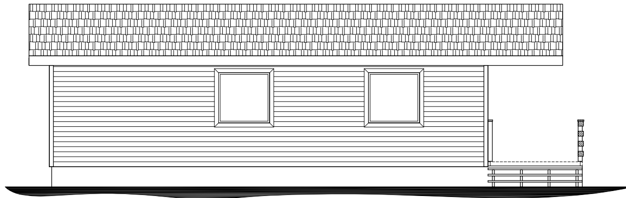
ELEWACJA BOCZNA
